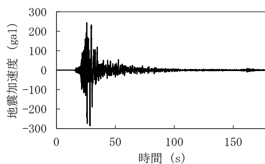
図 1 厚真町京町役場の加速度時刻歴 Fig.1 Acceleration time history of Atsuma Kyomachi Town Hall
